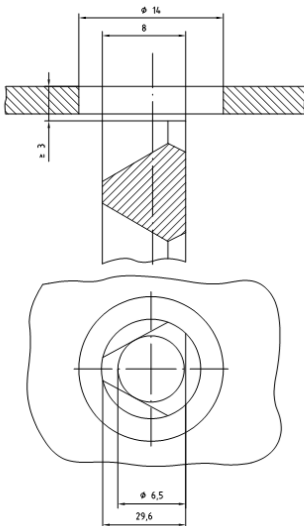
شکل ۷- مثلث قفل‌گشایی (به زیربند ۱-۲-۱۲ مراجعه شود)
